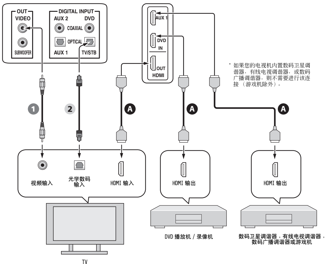
本机的后部面板
