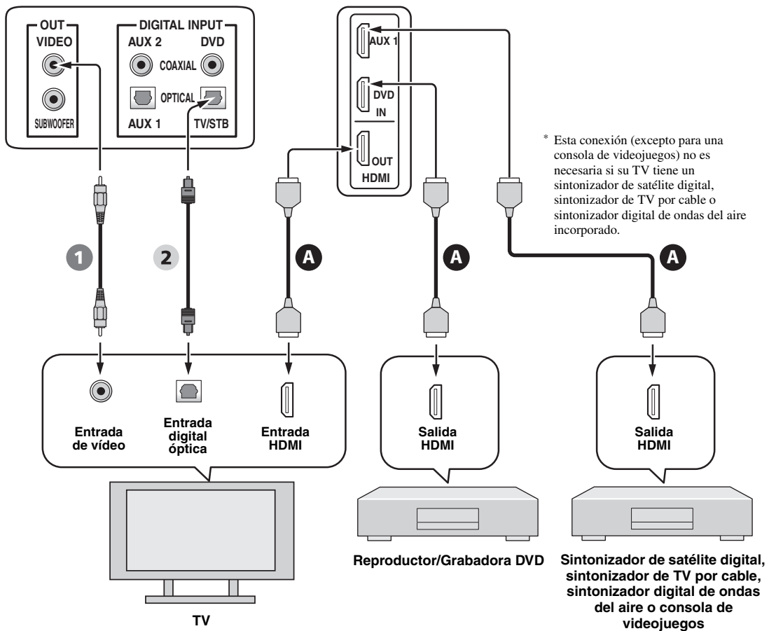
Panel trasero de esta unidad
